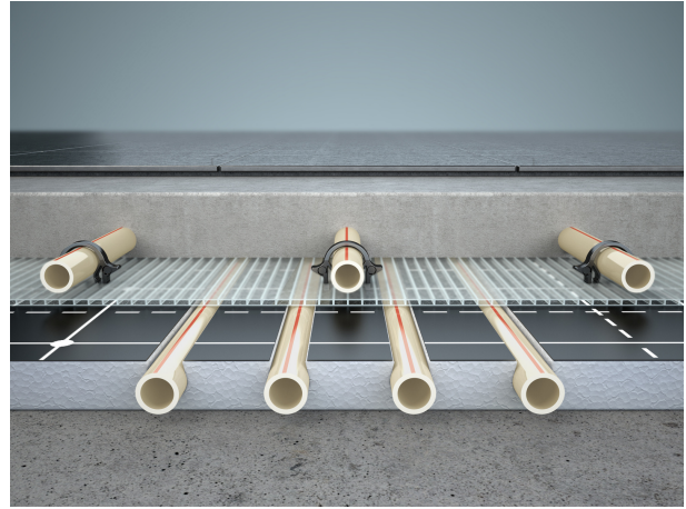
Bild 2: Anbindeleitung in Dämmebene in Kombination mit Tackersystem
